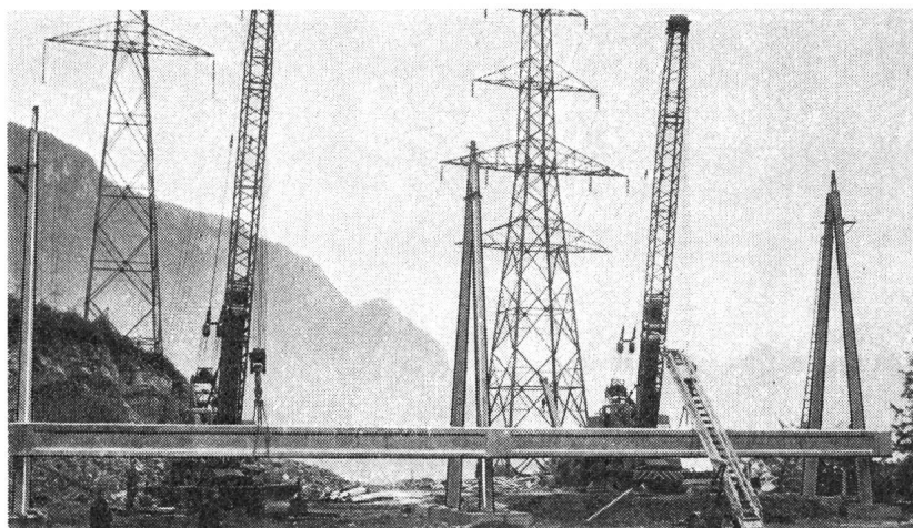
Travaux de montage du poste 220 kV. à Veytaux. (Force Motrice de l'Hongrin)
