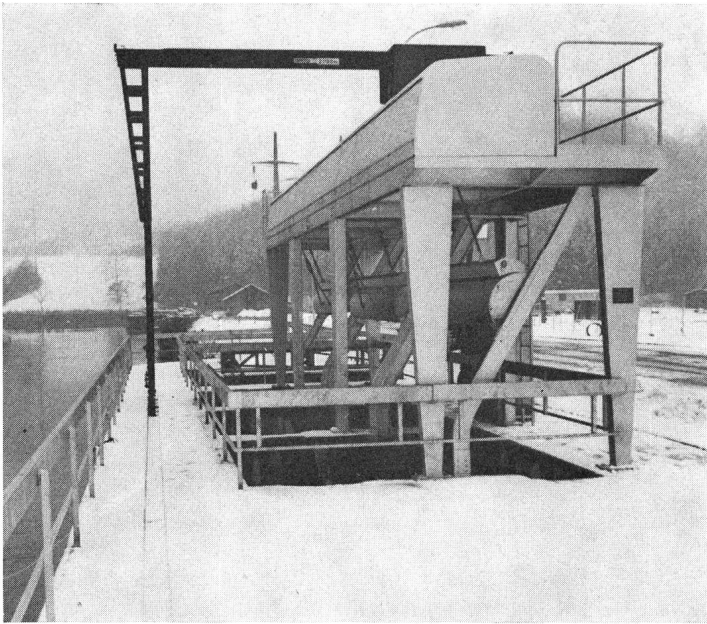
Kühlwasserfassung des Atomkraftwerks Beznau 3 Rechen- und 3 automatische, stationäre Rechen-Reinigungsmaschinen.
