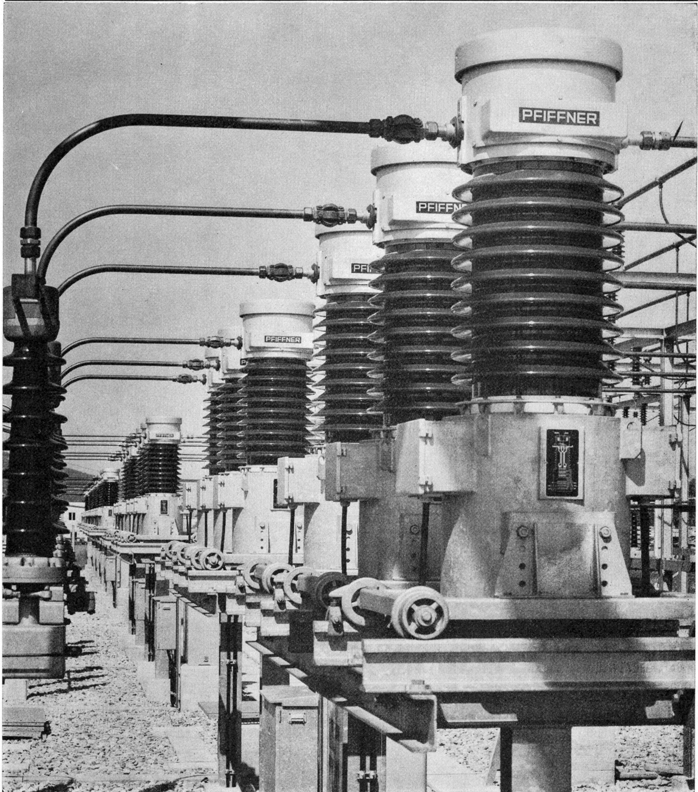
Messgruppen für max. Betriebsspannung 72,5 kV mit Ölisolation, vollständig geschlossene Bauart (Luft- und gasfreier Membranverschluss)
