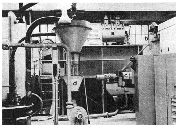
Fig. 1 Gelieranlage
