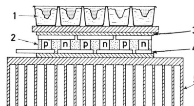
Fig. 22 Thermoelektrischer Kühler für Eisproduktion
