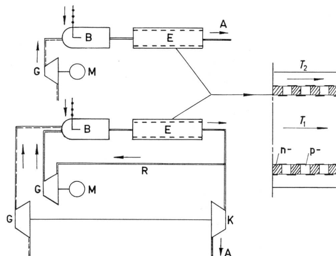
Fig. 21 Schema eines thermoelektrischen Energieerzeugers mittlerer Leistung
