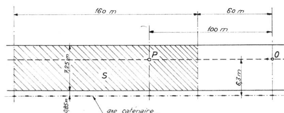
Fig. 8 Renseignements demandés au constructeur relatifs aux luminances P Luminance ponctuelle; S Luminance moyenne; O Observateur Hauteur d'observation = 1,50 m au-dessus du sol
