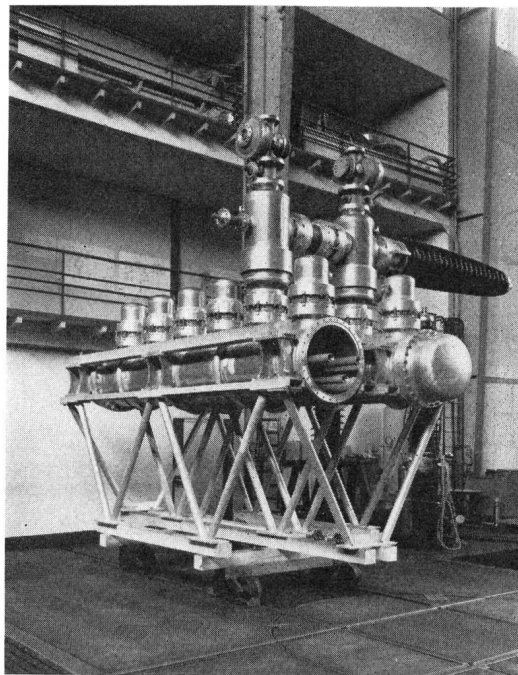
Fig. 6 Prototyp einer vollgekapelten Schaltanlage mit Druckgasisolation SF 6 für 245 kV
