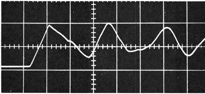
Fig. 8 In der Anordnung der Fig. 5a gemessene Einschwingspannung an der Versuchsleitung (vgl. Fig. 5b) Zeitmaßstab: 5-μs-Raster
