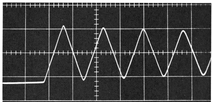
Fig. 7 In der Anordnung der Fig. 3c gemessene Einschwingspannung an der Versuchsleitung (vgl. Fig. 4) Zeitmaßstab: 5- \mu s -Raster
