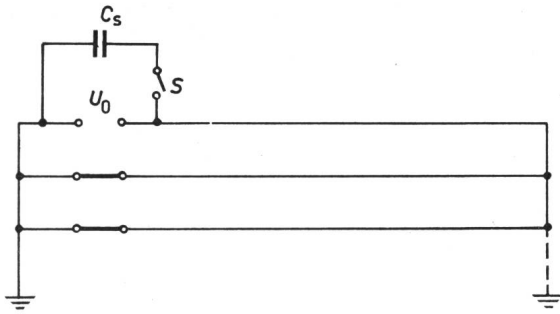
Fig. 6 Messanordnung
