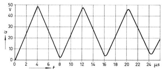
Fig. 14 Für die Versuchsleitung berechnete Einschwingspannung in der Anordnung gemäss Fig. 3c (vgl. Fig. 7) Erdleitfähigkeit K_E = 10^{-2} S/m
