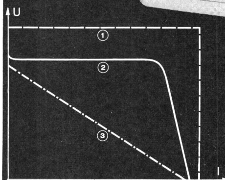
① IU-Kennlinie ② WESTAT-Kennlinie ③ W-Kennlinie
