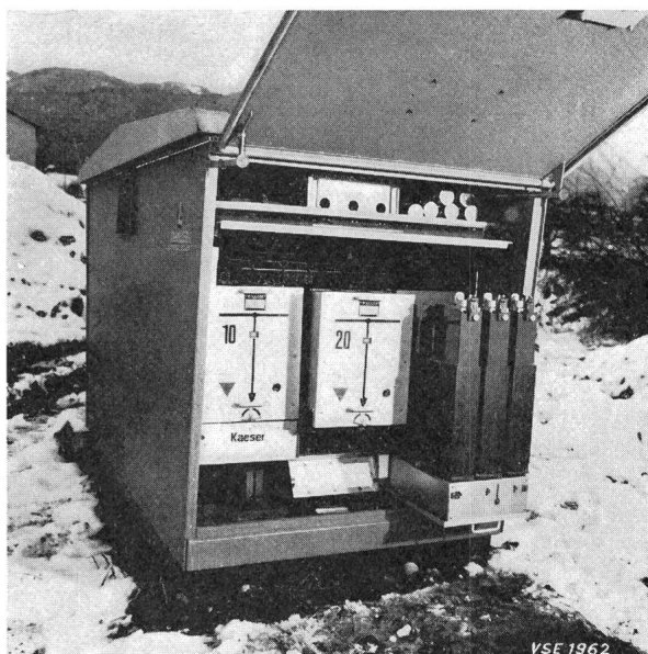
Fig. 2 Hochspannungs-Schalterschrank
