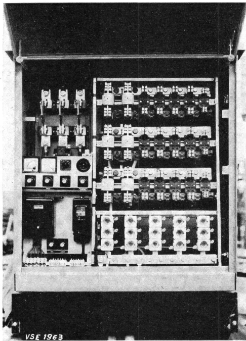
Fig. 3 Niederspannungs-Schaltschrank
