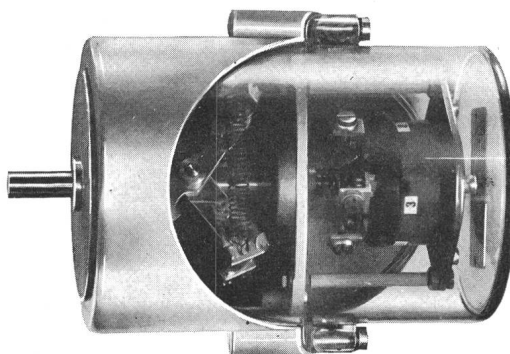
Fliehkraftschalter
