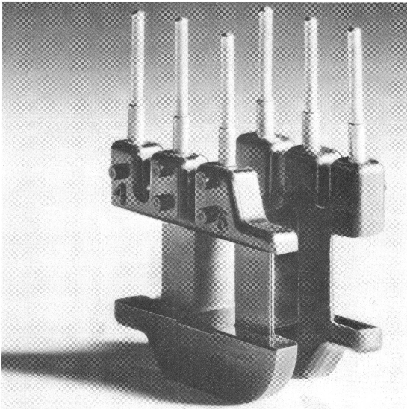
Trafo-Spulenkörper, stark vergrössert
