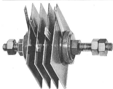
Selen Element
