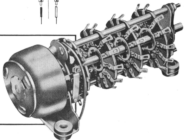
Typ 7S-8E
