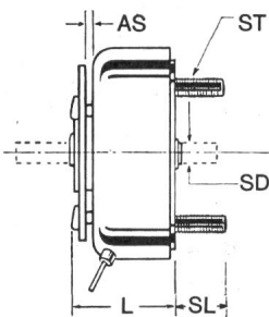
Typ 2E-6E
