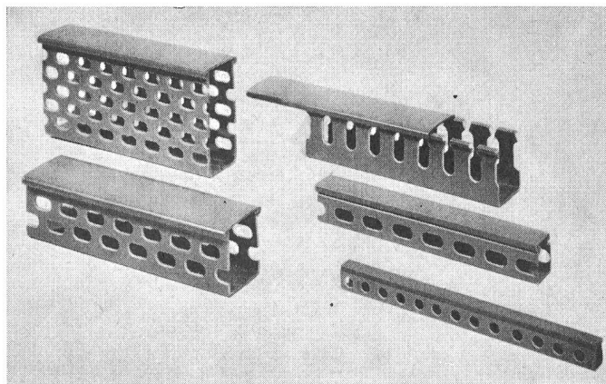
PVC-Kabelkanal mit oder ohne Perforierung Conduits de filerie en PVC rigide avec ou sans perforation
