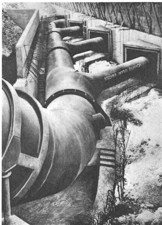
Kraftwerke Hinterrhein AG, Zentrale Sils, Verteilleitungen geschützt mit IMERIT LK-Mennig; Konstruktion der Firma Escher-Wyss AG, Zürich
