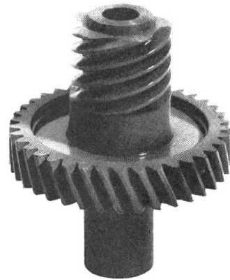
NYLON-ZAHNRÄDER
