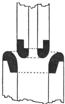
HOCHSPANNUNGS- LEISTUNGSSCHALTER
