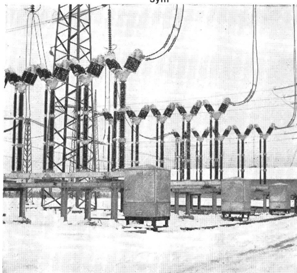
Ölarmes Leistungsschalter Typ HPF 516 in Kilförsen, Schweden
