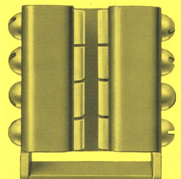
Federkontakt, Einheit in 3 Größen: Kontakt 250 A = zwei Fingerpaare Kontakt 400 A = drei Fingerpaare Kontakt 600 A = vier Fingerpaare
