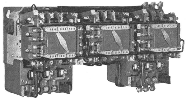
Polumschaltsschütze MPp 15/25 für Motoren in Dahlanderschaltung
