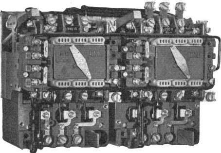
Polumschaltsschütze MWp 15/25 für Motoren mit 2 getrennten Wicklungen
