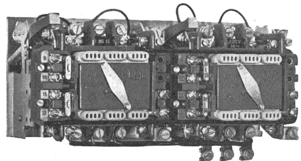
Umschaltsschütze MU 15/25
