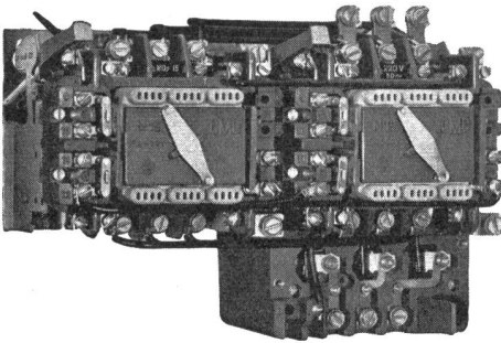
Drehrichtungsumschaltschütze MDp 15/25
