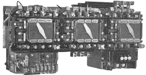
Sterndreieckschütze MSSp 40
