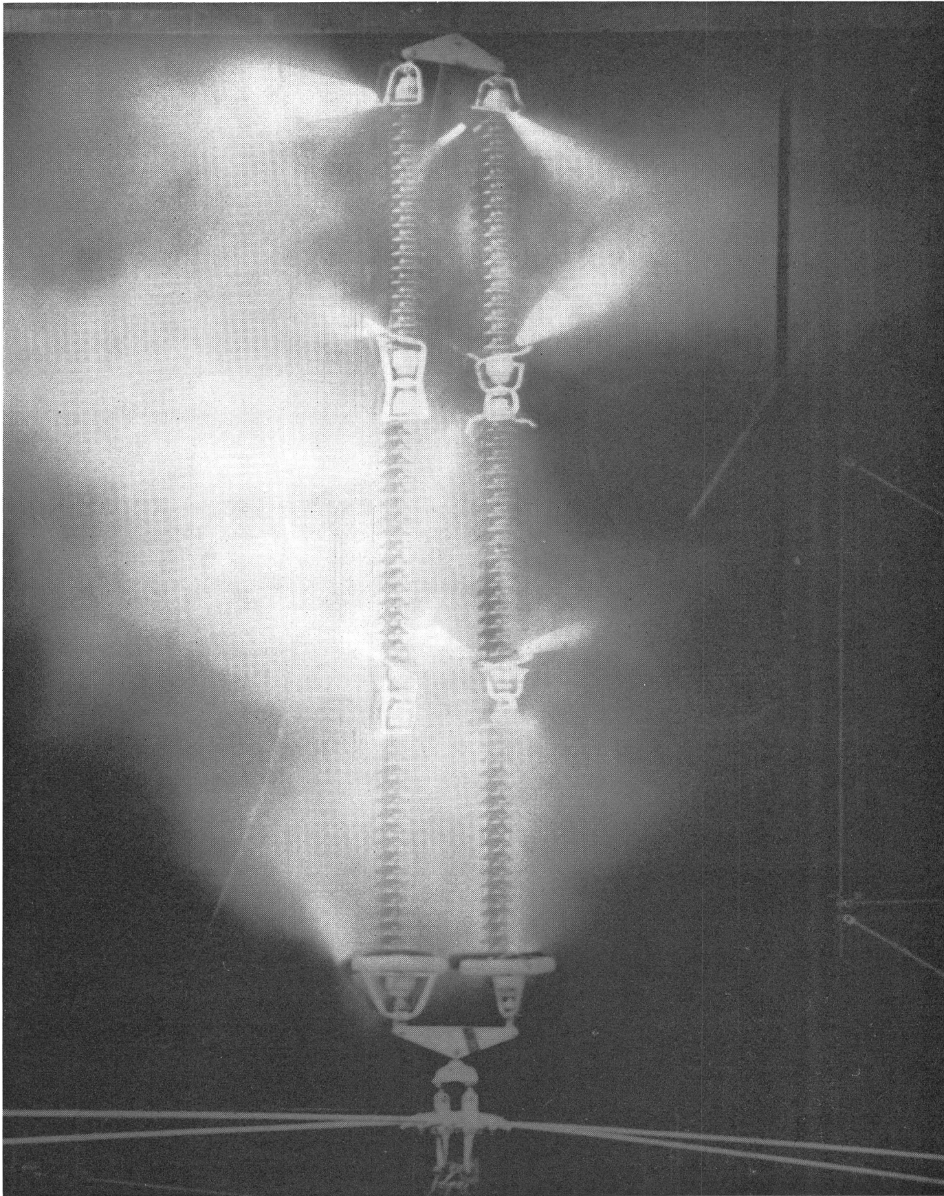
Hochstromversuch ausgeführt mit NORDEN LANGSTABISOLATOREN bei KEMA, Arnhem, Holland. Stromstärke 26.000 Amp. während 0,30 Sek.
