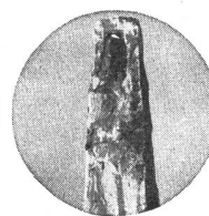
nach ca. 1400 Lötungen mit Normallot
