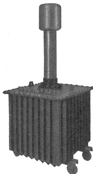
Prüftransformator 50/100/200 kV 40 kVA
