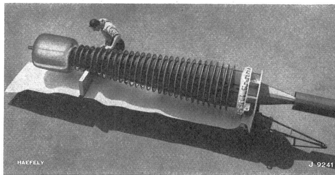
Transformator-Durchführung 420 kV
