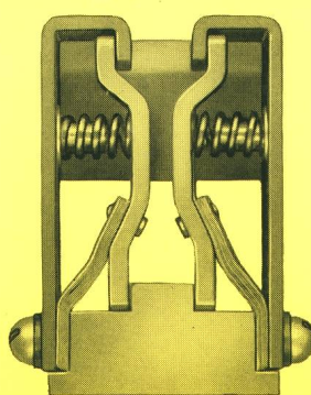
Spiralfedern rostfrei, vorgespannt
