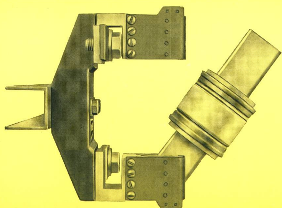
Kontakt Führungsblock für Sicherungen Müheloses Auswechseln der Patronen
