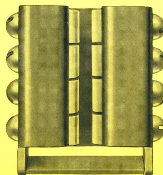
Federkontakt, Einheit in 3 Größen: Kontakt 250 A = zwei Fingerpaare Kontakt 400 A = drei Fingerpaare Kontakt 600 A = vier Fingerpaare
