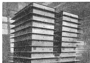
Teilstück einer Stollenauspan- zerung (Totalgewicht 80t)
