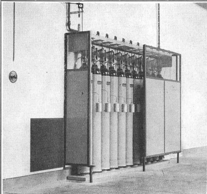
Unterstation La Coulouvrenière, Genf Automatischer Brandschutz mit Kohlendioxidregas
