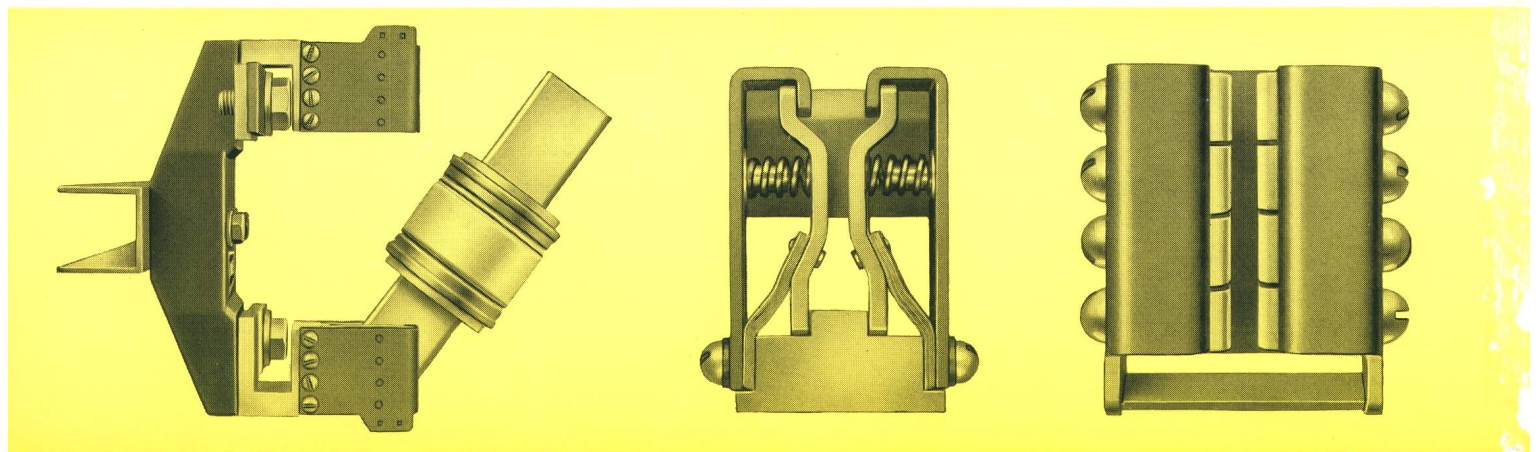
Kontakt Führungsblock für Sicherungen Müheloses Auswechseln der Patronen
