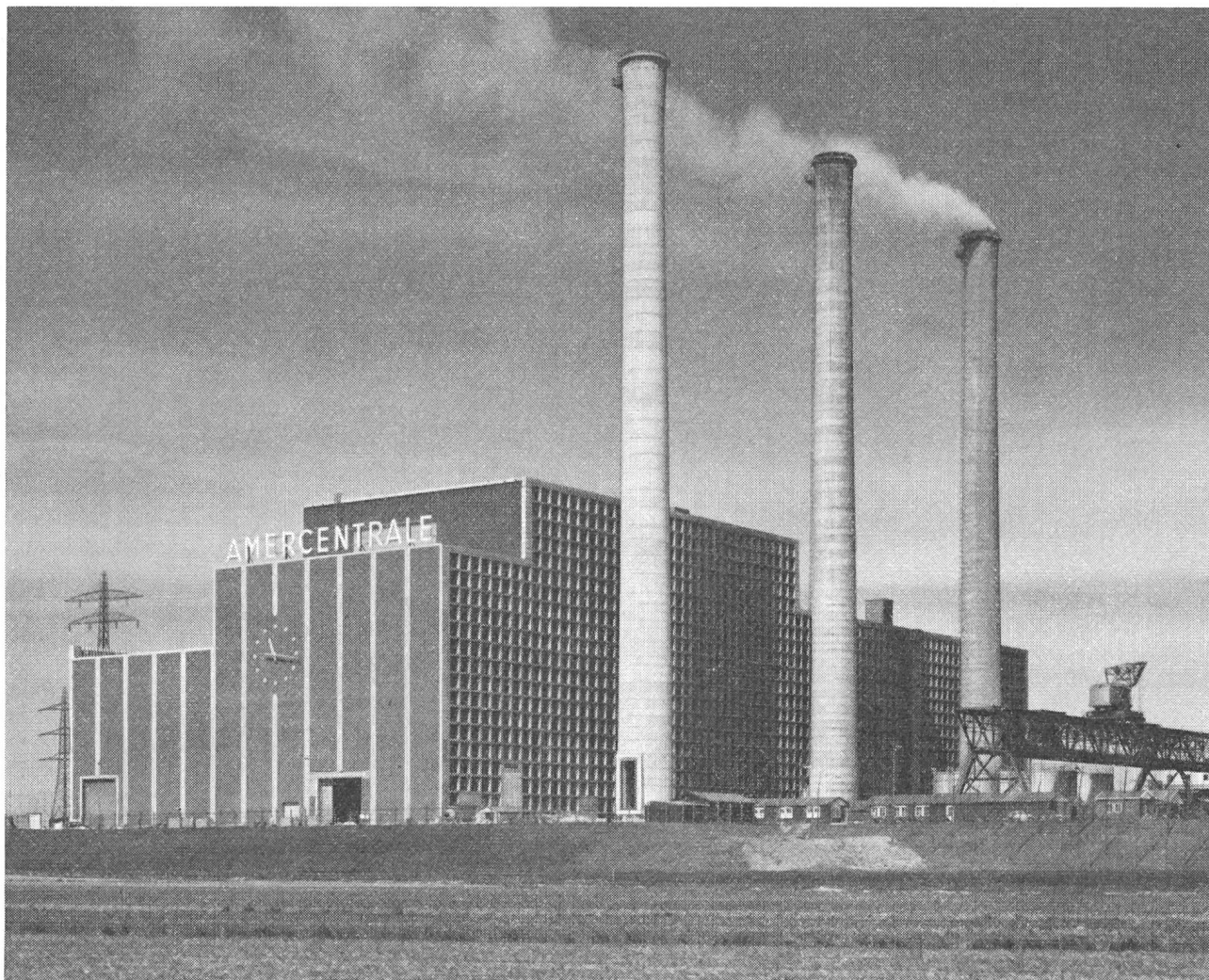
Thermisches Kraftwerk Amer der N. V. Provinciale Noordbrabantse Electriciteits-Maatschappij. 175 MW — Block ausgerüstet mit Schelde-Sulzer Einrohrdampferzeuger, 510 t/h, 180 atü, 570 °C.
