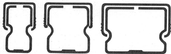
«TEHALIT»-Profile
