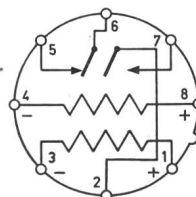
Schema 5 und 6
