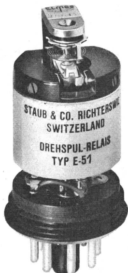
Typ ELMES 51 mit Plexiglashaube
