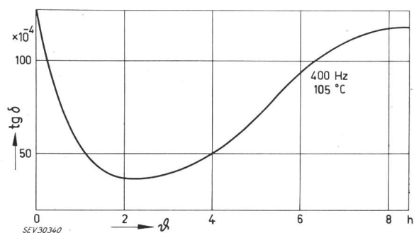
Fig. 3 Zeitverlauf einer Verlustfaktor-Messung \delta Zeit
