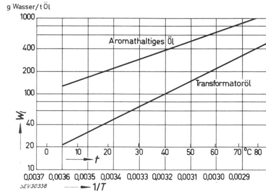
Fig. 1 Maximale Wasserlöslichkeit W_i in Funktion der Öltemperatur t T absolute Temperatur
