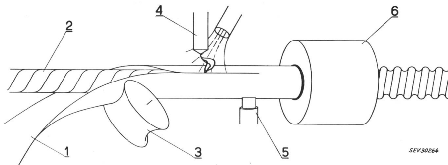
Fig. 3 Schematische Anfertigung des Wellmantels 1 Stahl- oder Kupferband; 2 Kabel; 3 Formwerkzeug; 4 Schweisselektrode; 5 Kohlebürste; 6 Welle
