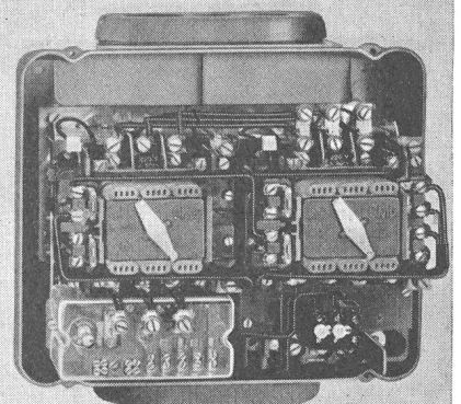
Sterndreieckschütz CMSp 25
