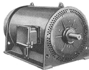
1050 kW/1480 U/min
