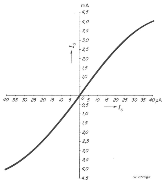
Fig. 9 Charakteristik eines Gegentaktsverstärkers I_a Ausgangsstrom; I_s Steuerstrom
