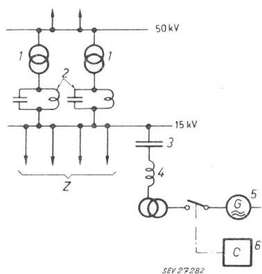
Fig. 2 Prinzipschema der Paralleleinspeisung mit Sperrkreis
