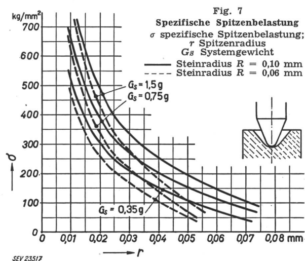
Fig. 7 zeigt einige statische, spezifische Lagerdrücke. Bei einem Systemgewicht von z. B. 0,75 g, einem Steinradius von 0,1 mm und einem Achsradius von 0,02 mm beträgt die spezifische Lagerbelastung 400 kg/mm 2 , also ein Wert, der im Maschinenbau nicht üblich ist.
