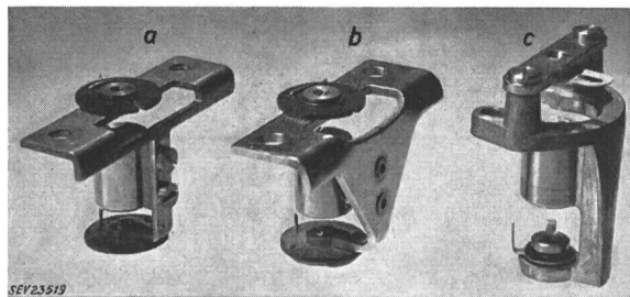
Fig. 9 Entwicklungsstufen des Messwerkstators a Stufe I: Messingstator, Kern geschraubt g^1 = 17,5 g b Stufe II: Messingstator, verstärkt, Kern genietet g^1 = 140 g c Stufe III: Spritzgußstator, Kern eingegossen g^1 = 300 g g^1 = Beschleunigungswert für 0,1 mm Einfederung der unteren Lagerstelle
