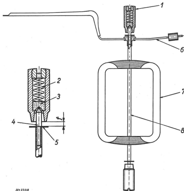
Fig. 8 Spitzenlagerung 1 Steinschraube; 2 Feder; 3 Stein; 4 Achsspitze; 5 Anschlagsscheibe; 6 Balancearm; 7 Rähmchen; 8 Rohrachse
