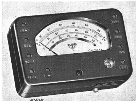
Fig. 12 Universalmessinstrument nach Fig. 11, geschlossen
