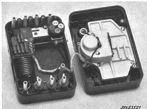
Fig. 11 Stossfestes Universalinstrument
