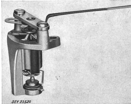
Fig. 10 Drehpulsmesswerk mit gefederten Spitzenlagern
