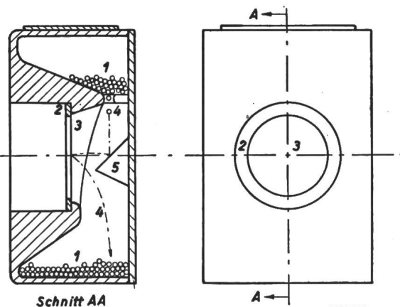
Fig. 11 Die Eichtonquelle des Technicum Neuchâtelois 1 Stahlkugel; 2 Ring; 3 Glimmermembran; 4 Bahn einer fallenden Kugel; 5 Prisma
