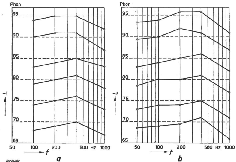
Fig. 8 Angezeigte Lautstärke als Funktion der Frequenz a Schalldruck sinusförmig b Schalldruck approximativ rechteckförmig L Lautstärke; f Frequenz; — angezeigte Werte; - - - - - eingestellte Werte
