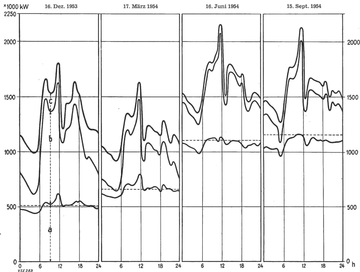
Fig. 10 Verlauf der Energieerzeugung an Mittwochen
