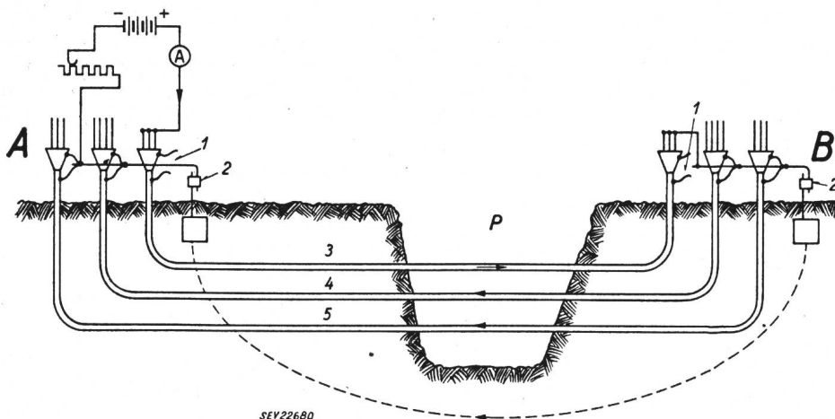
Exemple d'identification d'un câble tripolaire haute tension en parallèle avec deux autres câbles en service
