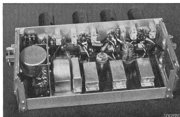
Fig. 2 Verstärkerhälfte
