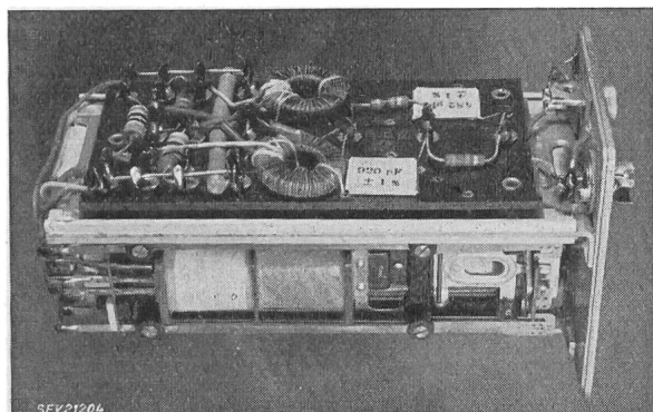
Fig. 3 Temperaturkorrektor
