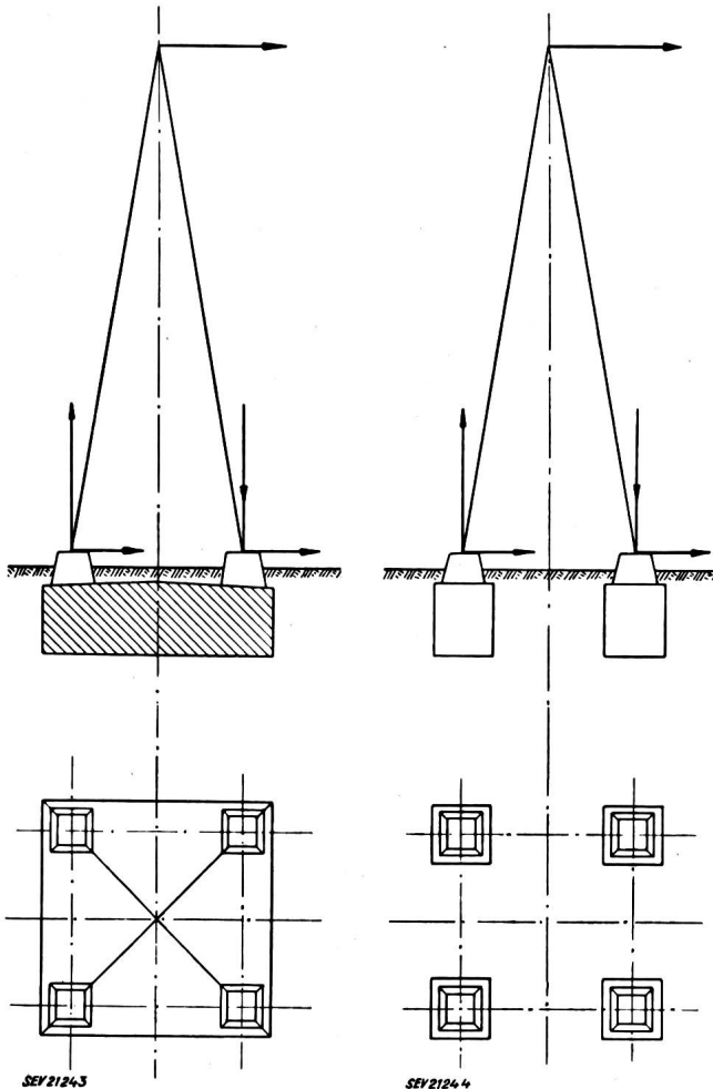
Fig. 2 Blockfundament
