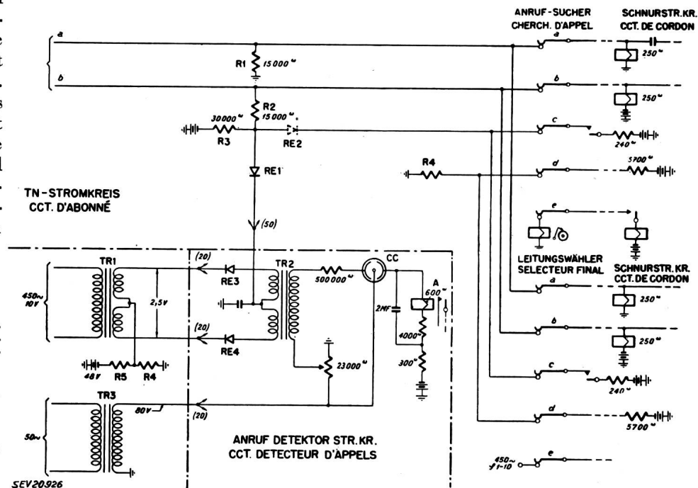
Fig. 6 Circuit d'abonné et détecteur d'appels R_1 , R_2 , R_3 résistances du diviseur de tension; RE_1 redresseur; R_4 résistance caractéristique de la ligne; TR_2 transformateur; RE_3 , RE_4 redresseurs; CC tube à cathode froide; A relais de contrôle TR_1 transformateur, 450 p/s; TR_3 transformateur, 50 p/s
