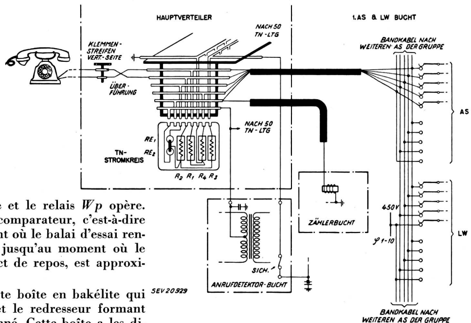
Fig. 9 Schéma de la réglette de raccordement du distributeur principal
