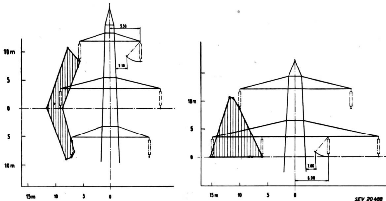
Vergleich des beanspruchten Leiterraumes von zweisträngigen 380-kV-Leitungen
