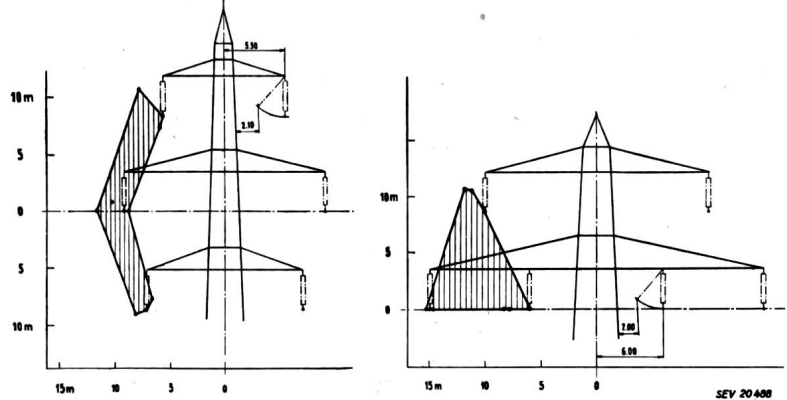
Fig. 4 Vergleich des beanspruchten Leiterraumes von zweisträngigen 380-kV-Leitungen links: Tannenbaumordnung; rechts: Donaumastbild, hauptsächlich in Deutschland angewendet, in der Schweiz auf einer Teilstrecke der Leitung Amsteg-Mettlen
