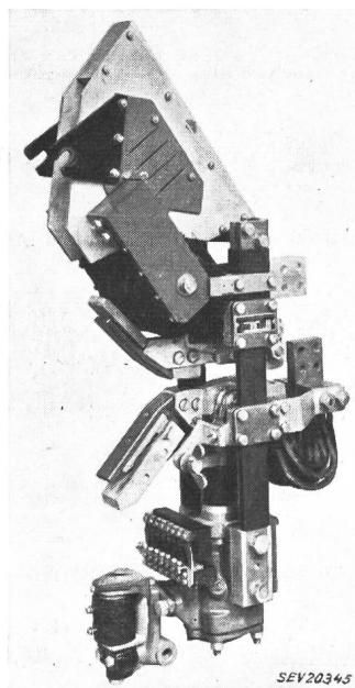
Fig. 4 Hüpfen für Stromstärken bis 2600 A
