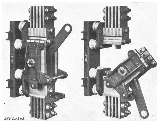
Fig. 2 Trenner für grosse Stromstärken
