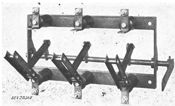
Fig. 1 Einfacher Trenner
