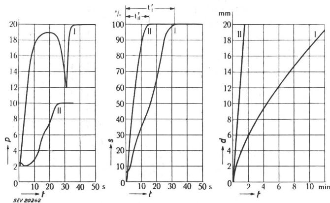
Fig. 12 Kunstharzpressen
