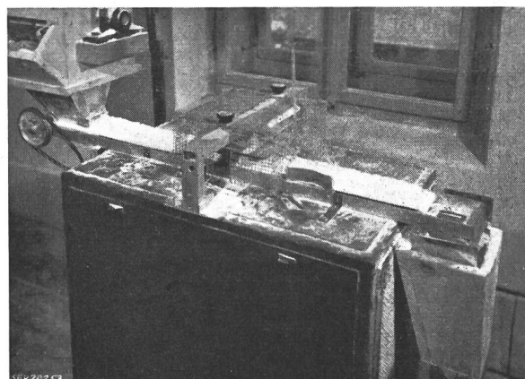
Fig. 23 Versuchsanlage zur Mehlsterilisierung mit Hochfrequenz-Energie im Durchlaufverfahren
