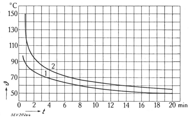
Fig. 14 Heissverleimung von Holz
