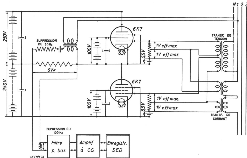
Fig. 4 Multiplicateur électronique pour la mesure de la puissance
