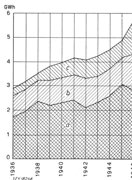
Fig. 3 Portugiesische Elektrizitätserzeugung a Wärmekraftwerke b Laufwerke c Speicherwerke } Wasserkraftwerke
