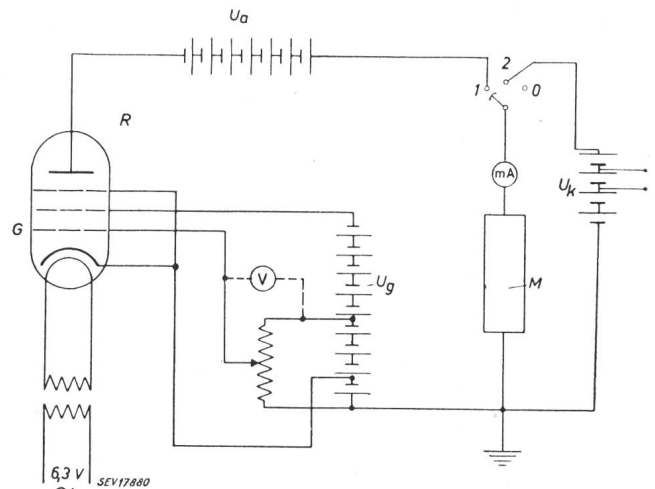
Fig. 3 Schaltbild der röhrengesteuerten Einrichtung zur Konstanzhaltung von Modellströmen und Modellspannungen R Pentode mit hohem Innenwiderstand; G Steuergitter; M Modell; U_a Anodenspannung; U_g Gitterspannung; U_k konstante Spannungsquelle mit verschiedenen Anzapfungen
