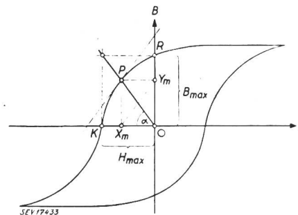
Fig. 2 Magnetisierungskurven
