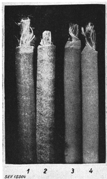
Fig. 4 Câbles isolés exposés 1 et 2 heures aux effets de l'ozone 1 et 2 Caoutchouc naturel 3 et 4 Thermoplaste à base de chlorure de polyvinyle
