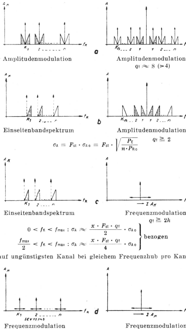
Fig. 7 Frequenzmultiplex-Einträgersysteme mit einer einzigen gemeinsamen Modulation links: Kanalträgerspektrum rechts daneben: zugehöriges UKW-Träger-Spektrum (Symbole siehe in der Legende zu Fig. 8)
