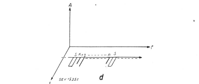
d Trägertastung mit vormodulierten Impulsen Frequenzmodulation (z. B. Amplitudenmodulation)
