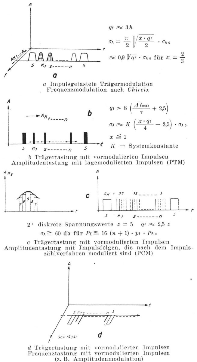
Fig. 11 Zeitmultiplex-Systeme \Delta f_{\max} maximaler Zeithub eines Impulses; \tau Impulsdauer; z Anzahl der Impulse pro Impulsfolge (Zahlengruppe) Übrige Symbole siehe in der Legende zu Fig. 8
