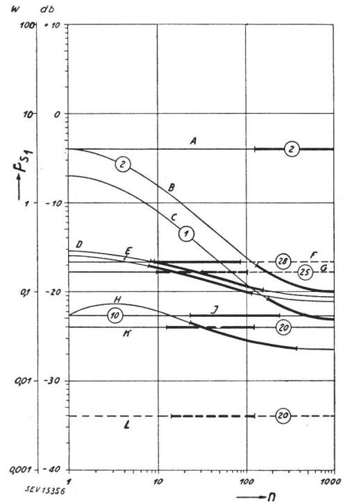
Fig. 15 Erforderliche mittlere Senderleistung pro Kanal mit Rücksicht auf das reine Empfängerrauschen Voraussetzungen siehe Text. Die eingekreisten Zahlen bedeuten den Frequenzbandfaktor q_f , während die dick ausgezogenen Kurventeile jeweils einen Bereich von 1...10 MHz Bandbreite umfassen. n Anzahl der Kanäle; P_{S1} mittlere Senderleistung pro Kanal
