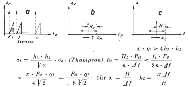
Fig. 8 Frequenzmultiplex-Einträgersysteme mit doppelter gemeinsamer Modulation a Kanalträgerspektrum (Einseitenband-Spektrum) (Index K ) b Zwischenträger (Frequenzmodulation) (Index Z ) c UKW-Träger (Frequenzmodulation) \Delta f Bandbreite; F_{st} Verbesserungsfaktor infolge statistischer Überlagerung der Gesprächsamplituden nach Fig. 14; H Frequenzhub; h Hubverhältnis (max. Frequenzhub/max. Modulationsfrequenz); K_{1..n} niederfrequente Nachrichtenkanäle; n Anzahl der Nachrichtenkanäle; P_E , P_{R0} Signal- bzw. Rauschleistung vor dem nichtlinearen Glied des Empfängers; q_i Frequenzbandfaktor; \sigma_A Verhältnis Signal/Geräusch in einem niederfrequenten Empfangskanal; \sigma_{A0} bezieht sich auf Zweiseitenband-Amplitudenmodulation; x Frequenzbandausnutzung (Frequenzhub/Bandbreite des Empfängers)
