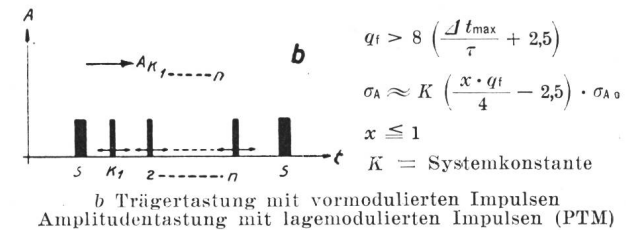
b Trägertastung mit vormodulierten Impulsen Amplitudentastung mit lagemodulierten Impulsen (PTM)
