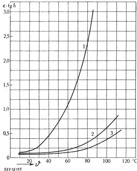
Fig. 1 Temperaturabhängigkeit der Verlustziffer verschiedener Nutsisolationen 1 Glimmer mit Schellack geklebt; 2 Glimmer mit Asphaltlack geklebt; 3 Ausführung nach verbessertem Fabrikationsverfahren
