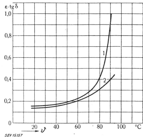
Fig. 3 Temperaturabhängigkeit der Verlustziffer einer Isolation mit grossen dielektrischen Verlusten 1 Verlustziffer, gemessen vor dem Dauerversuch (Fig. 2); 2 Verlustziffer, gemessen nach dem zweiten Dauerversuch (Fig. 2)
