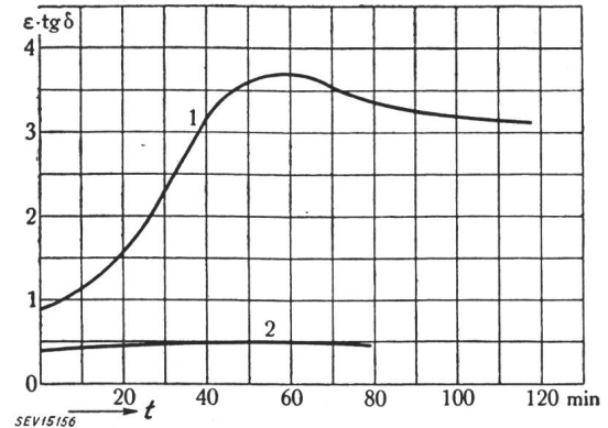
Fig. 2 Dauerversuch an einer Isolation mit grossen dielektrischen Verlusten Verlustziffer in Funktion der Zeit 1 Erster Versuch bei konstanter Wechselspannung von 90 kV; 2 Zweiter Versuch bei derselben Spannung Beide Versuche bei 90°C am geerdeten Messbelag
