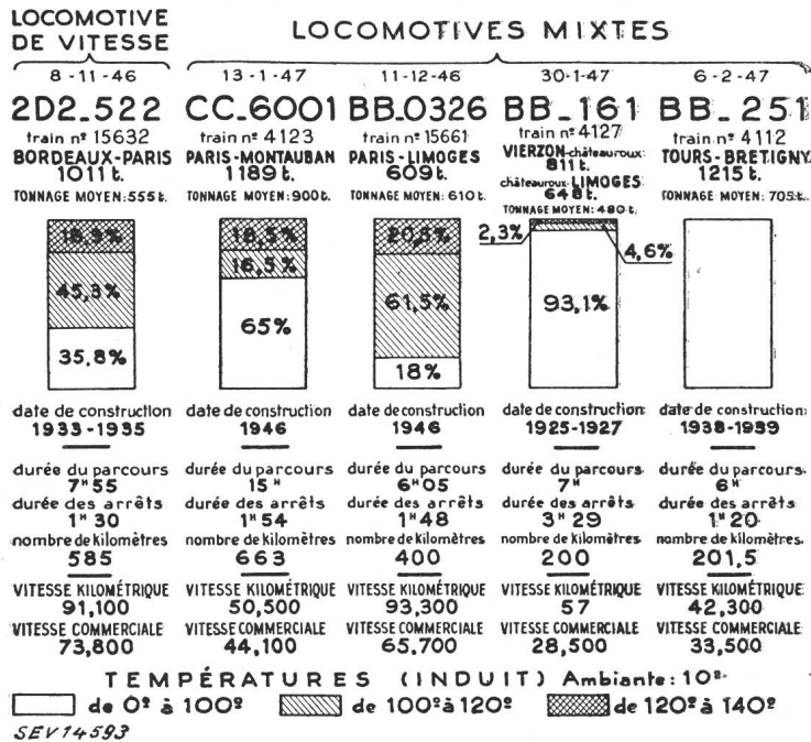
Températures relevées en service sur la SNCF
