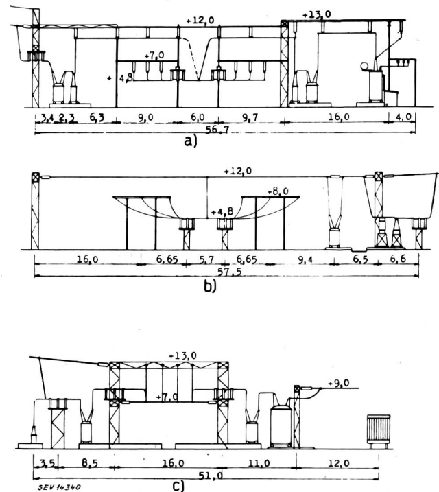
Fig. 5 Schweizerische Freiluftanlagen a) Hochbauform 1922 b) Halbhochbau 1932 c) aufgelöster Gitterträgerbau 1926
