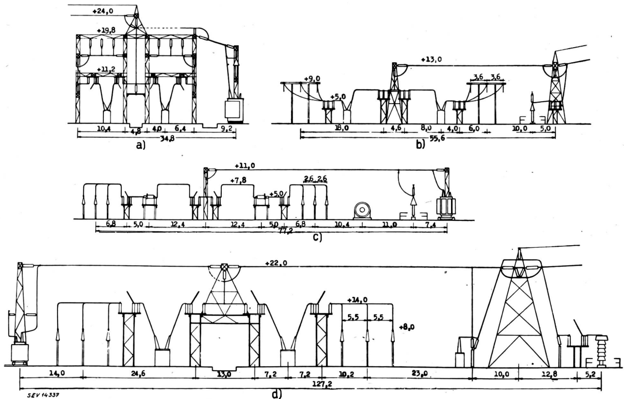
Fig. 2 Amerikanische Freiluftanlagen
