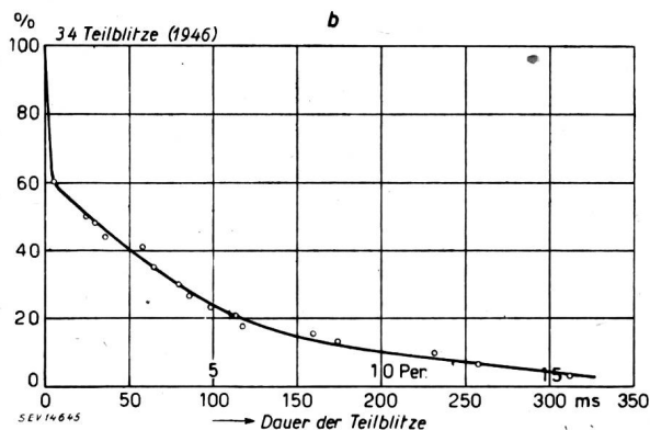
Fig. 15 Häufigkeit verschiedener Dauer der Teilblitze a Aus 56 Teilblitzen (1943...1946) b Aus 34 Teilblitzen (1946)
